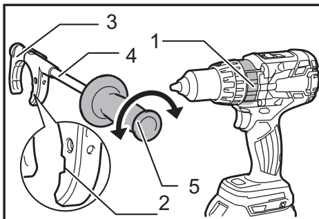
► 1. Saillie 2. Rainure 3. Bras 4. Tige de la poignée 5. Poignée latérale
