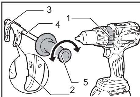
► 1. Protrusion 2. Groove 3. Arm 4. Grip pole 5. Side grip
