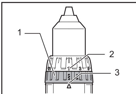
► 1. Bague de changement de mode d'action 2. Graduation 3. Flèche
