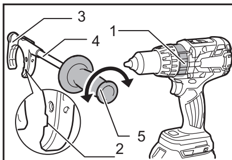
► 1. Protuberancia 2. Ranura 3. Brazo 4. Vara de sujeción 5. Empuñadura lateral de mango
