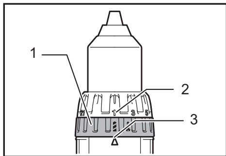
► 1. Anillo de cambio del modo de acción 2. Graduación 3. Flecha
